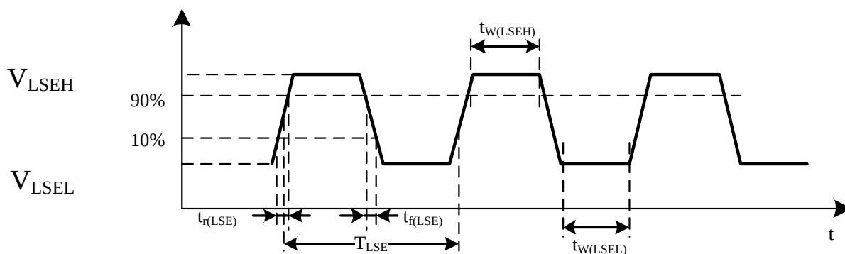
图 12 低速外部时钟源交流时序图
