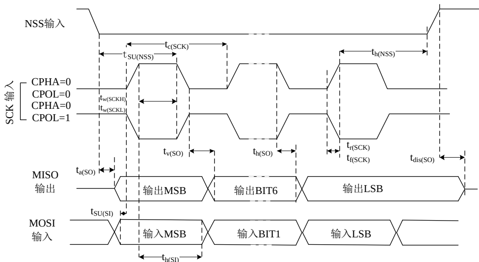
图 21 SPI 时序图-从模式和 CPHA=0
