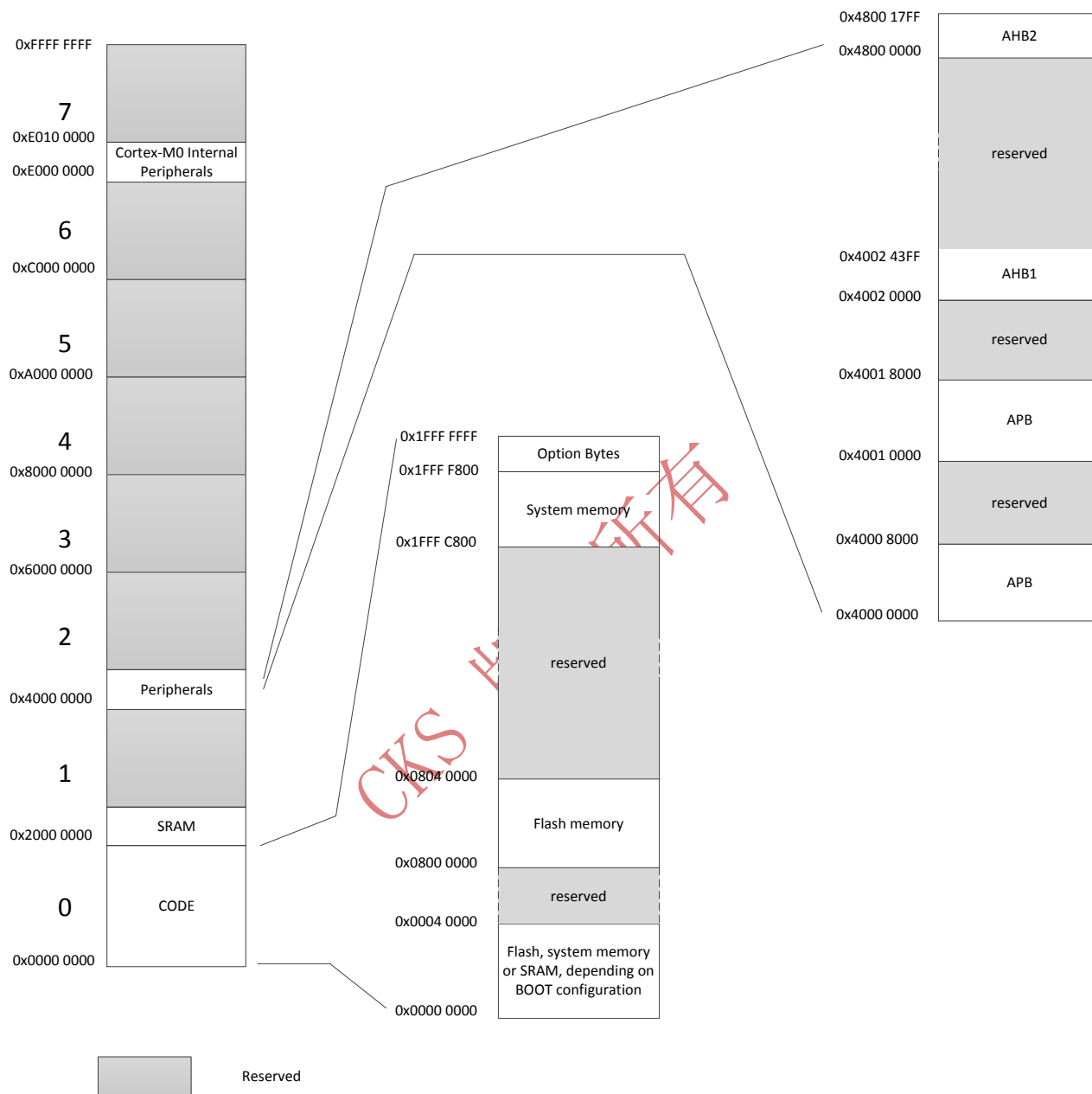
图 6 CKS32F030xx 内存映射
