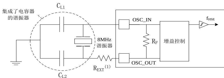
图 13 使用 8MHz 晶体的典型应用
