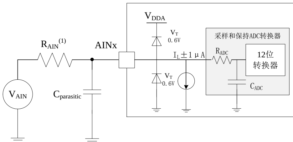
图 20 使用 ADC 典型的连接图
