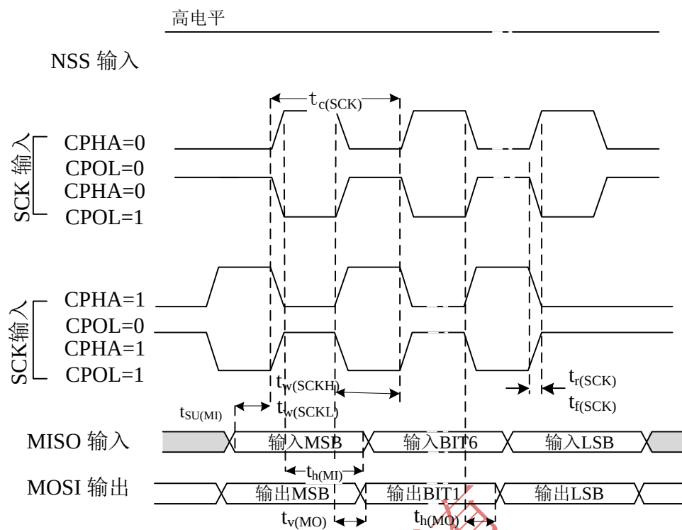
图 23 SPI 时序图-主模式 (1)
