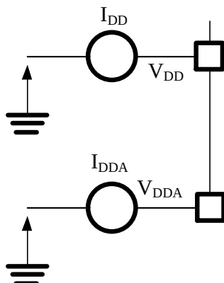
图 10 电流消耗测量方案
