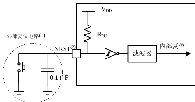
图 18 建议的 NRST 引脚保护
