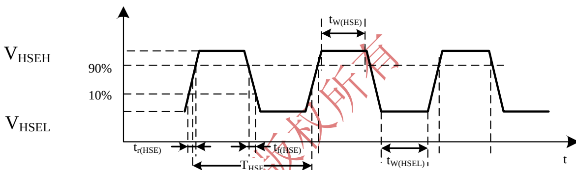
图 11 高速外部时钟源交流时序图
