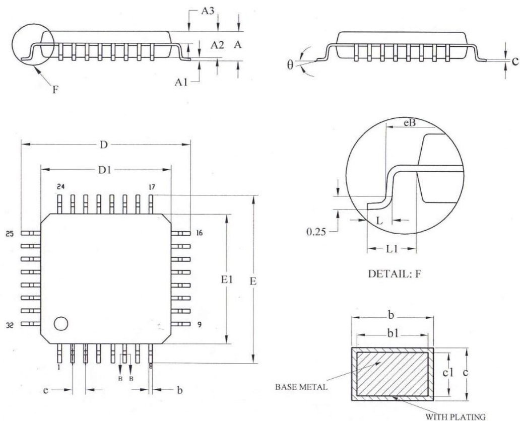
图 26 LQFP32-7x7 mm, 32 脚低剖面方形扁平封装图
