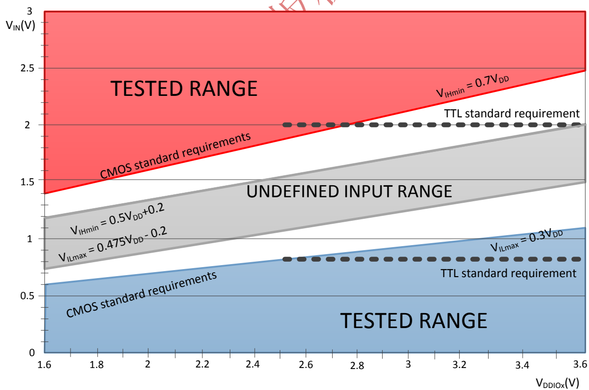
图 16 5V 容忍(FT 和 FTf)的 I/O 输入特性
