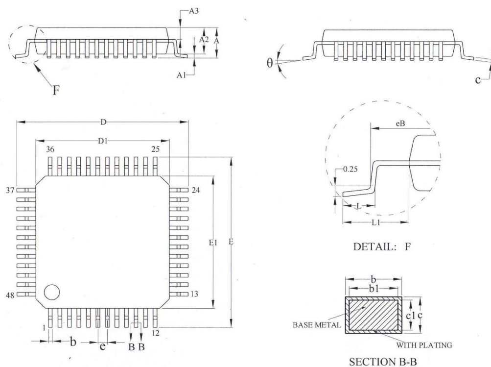
图 24 LQFP48-7x7mm, 48 脚低剖面方形扁平封装图
