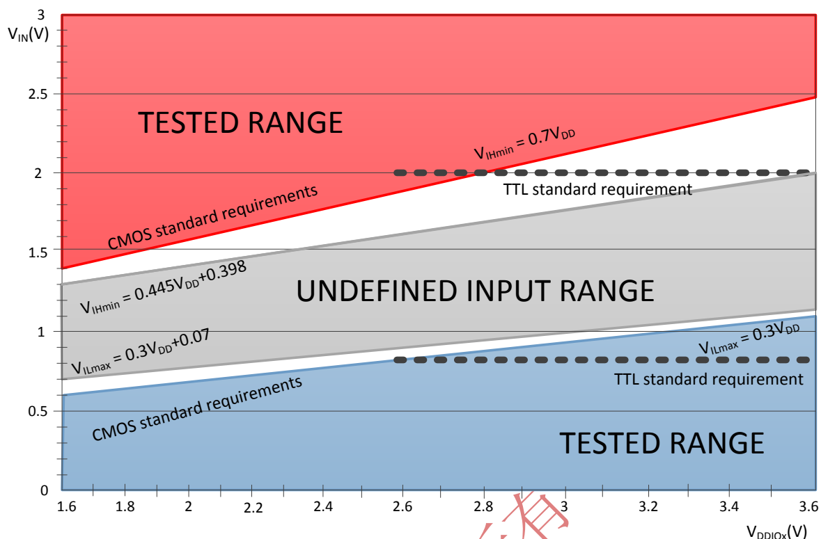
图 15 TC 和 TTa 的 I/O 口输入特性
