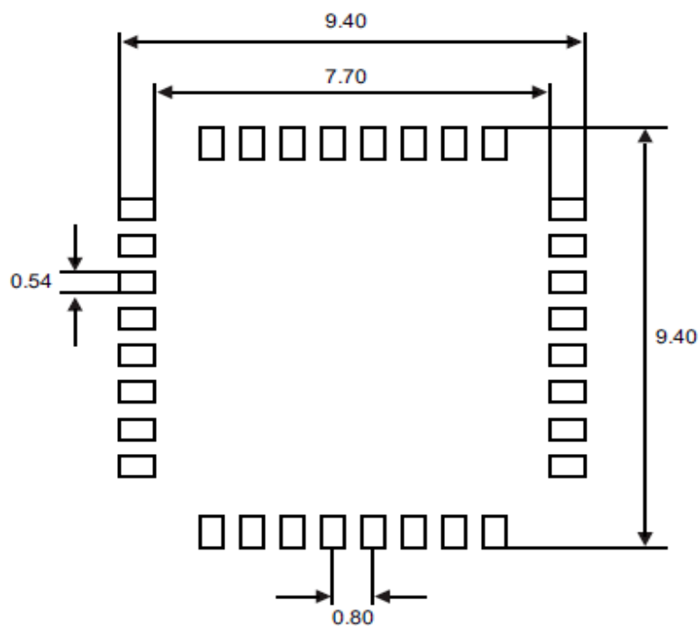
图 27 LQFP32 推荐封装
