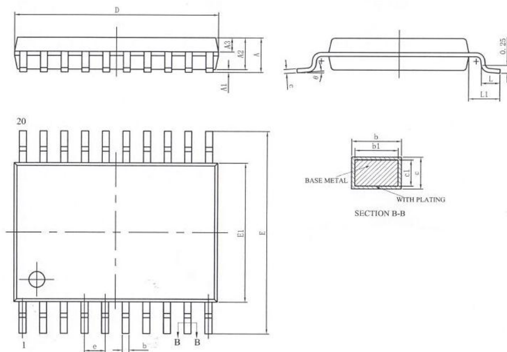
图 28 TSSOP20-20 脚薄细封装图
