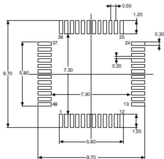
图 25 LQFP48 推荐封装
